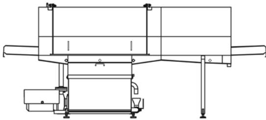
Modulare Mehr-Zonen Tunnelwaschmaschinen, Länge der Module 1750 mm, Transportbreite von maximal 60 cm.
